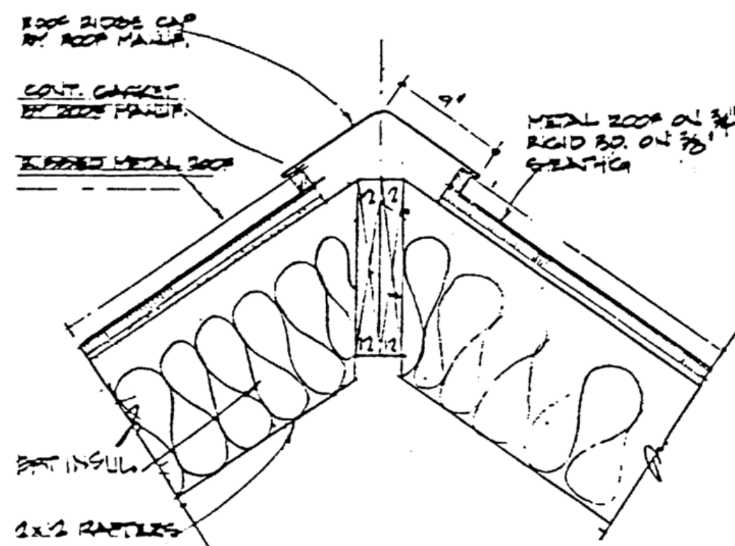
Ridge Detail #1 / D1 N.T.S.
