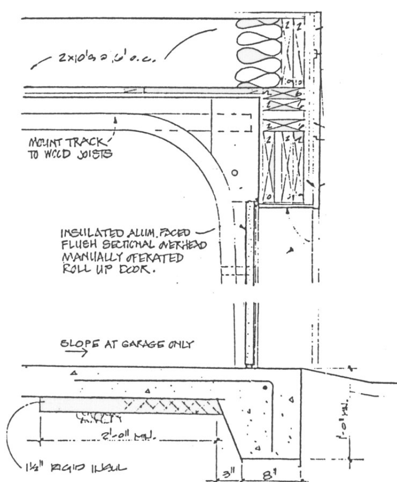
Garage Door Detail #6 / D3 N.T.S.
