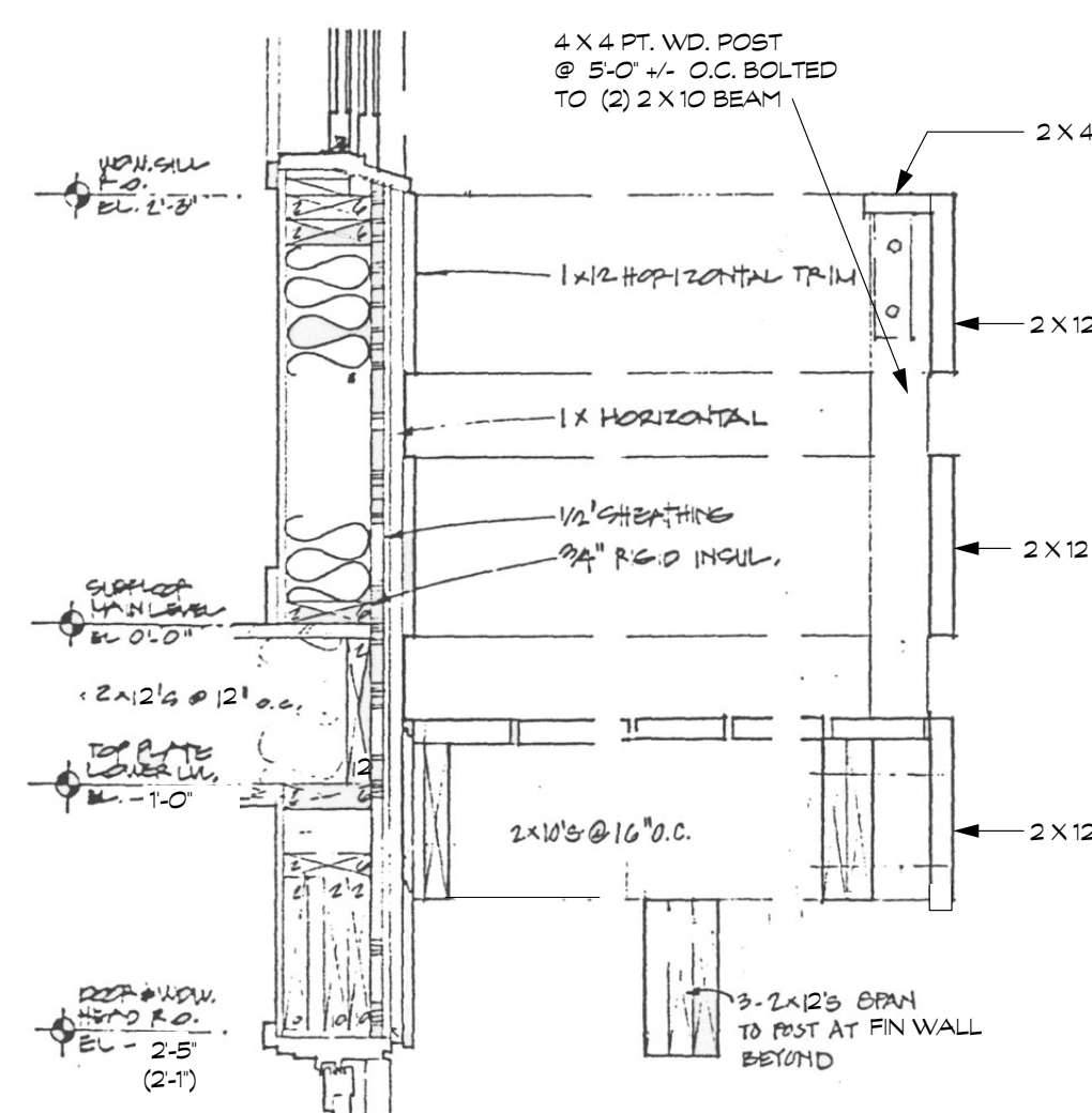
Exterior Rail #10 / D6 N.T.S.
