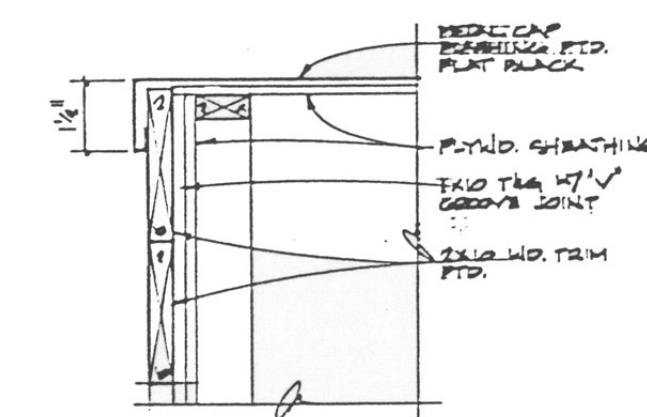
Chimney Cap #11 / D6 N.T.S.
