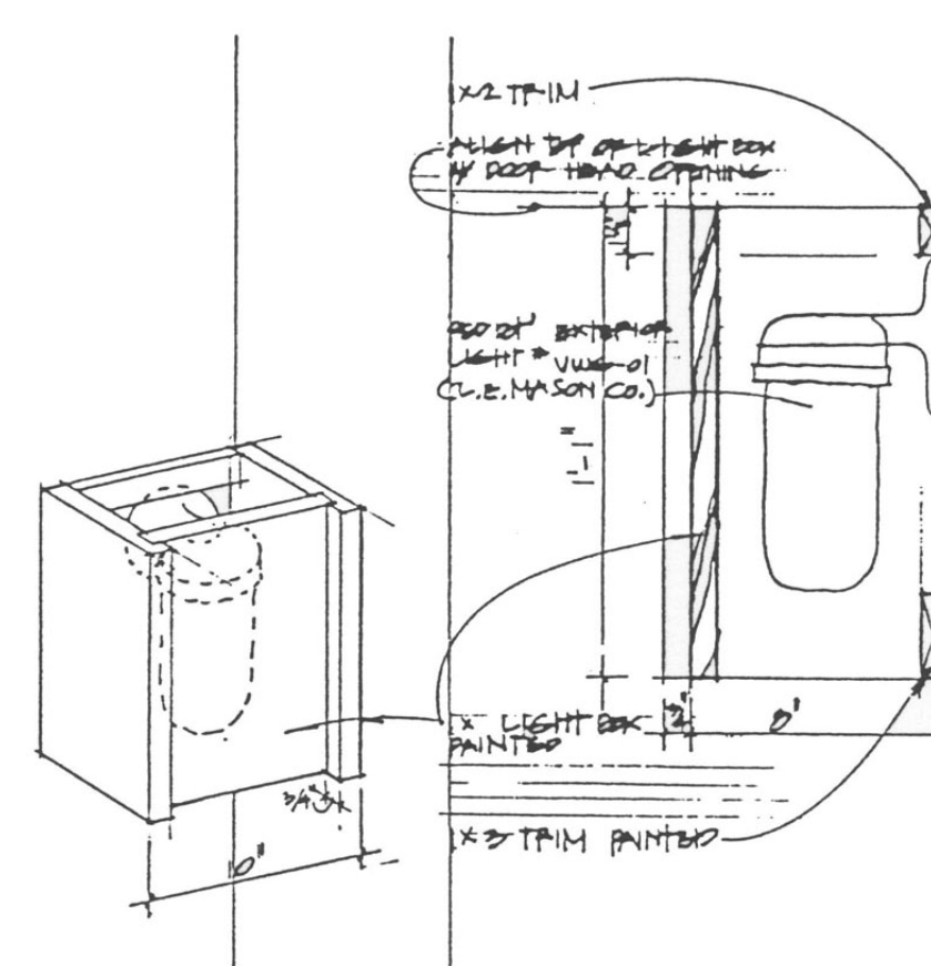
Exterior Light Box Detail #4 / D2 N.T.S.
