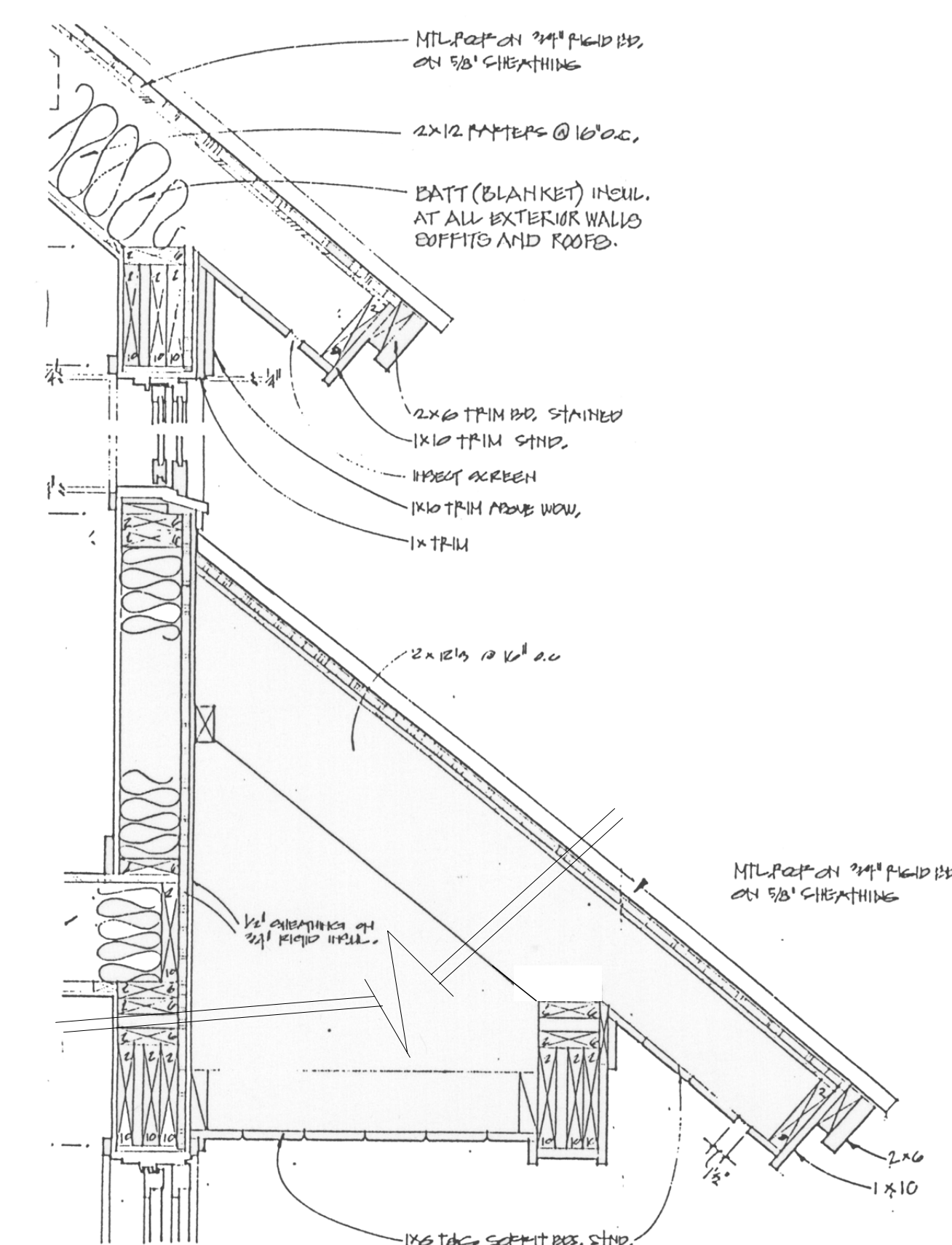
Eaves Detail #27 / D16 N.T.S.
