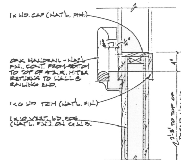
Rail (optional) Detail #7 / D4 N.T.S.
