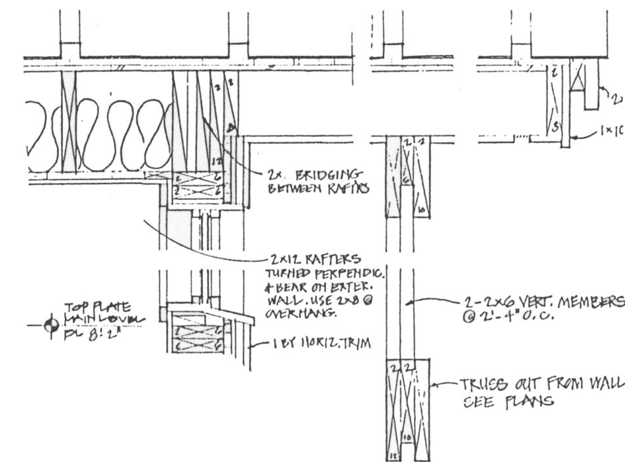
Truss Detail #5 / D3 N.T.S.
