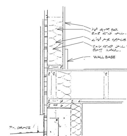
Side Wall #18 / D11 N.T.S.
