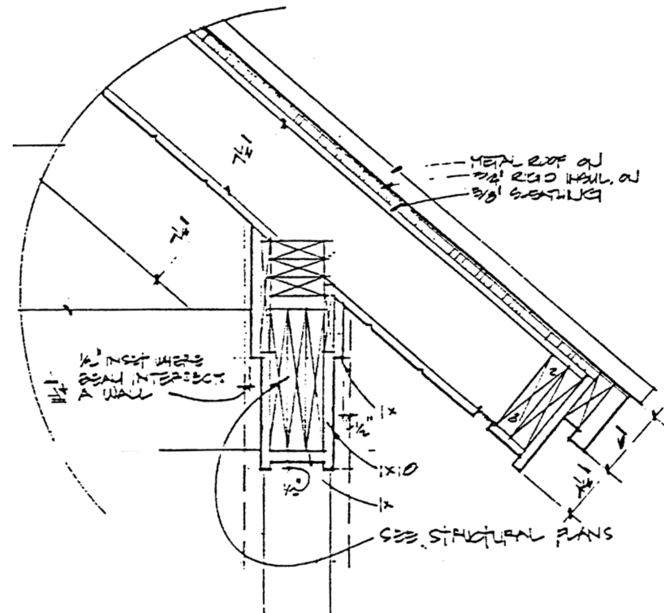
Encased Beam Detail #2 / D1 N.T.S.
