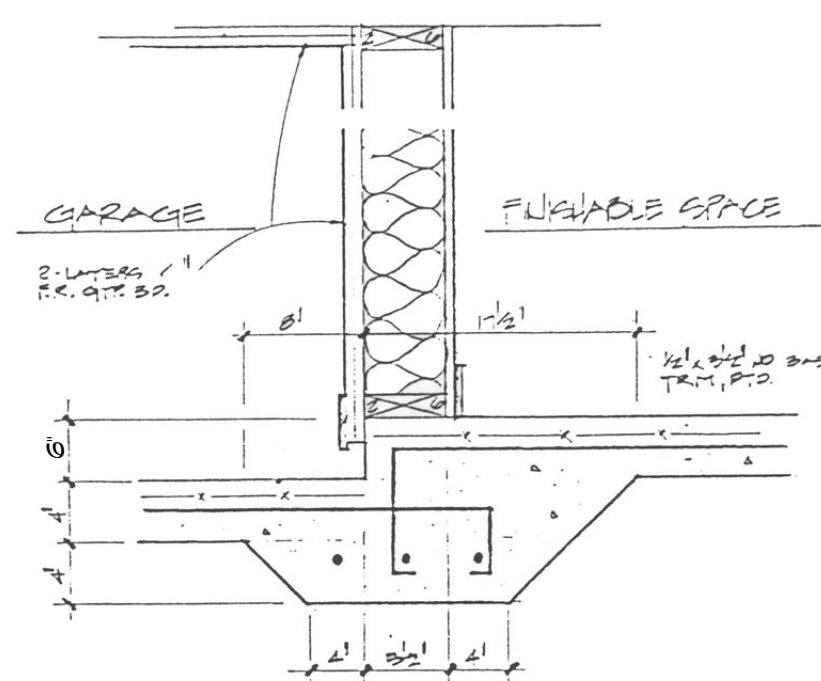
Garage Wall #13 / D7 N.T.S.
