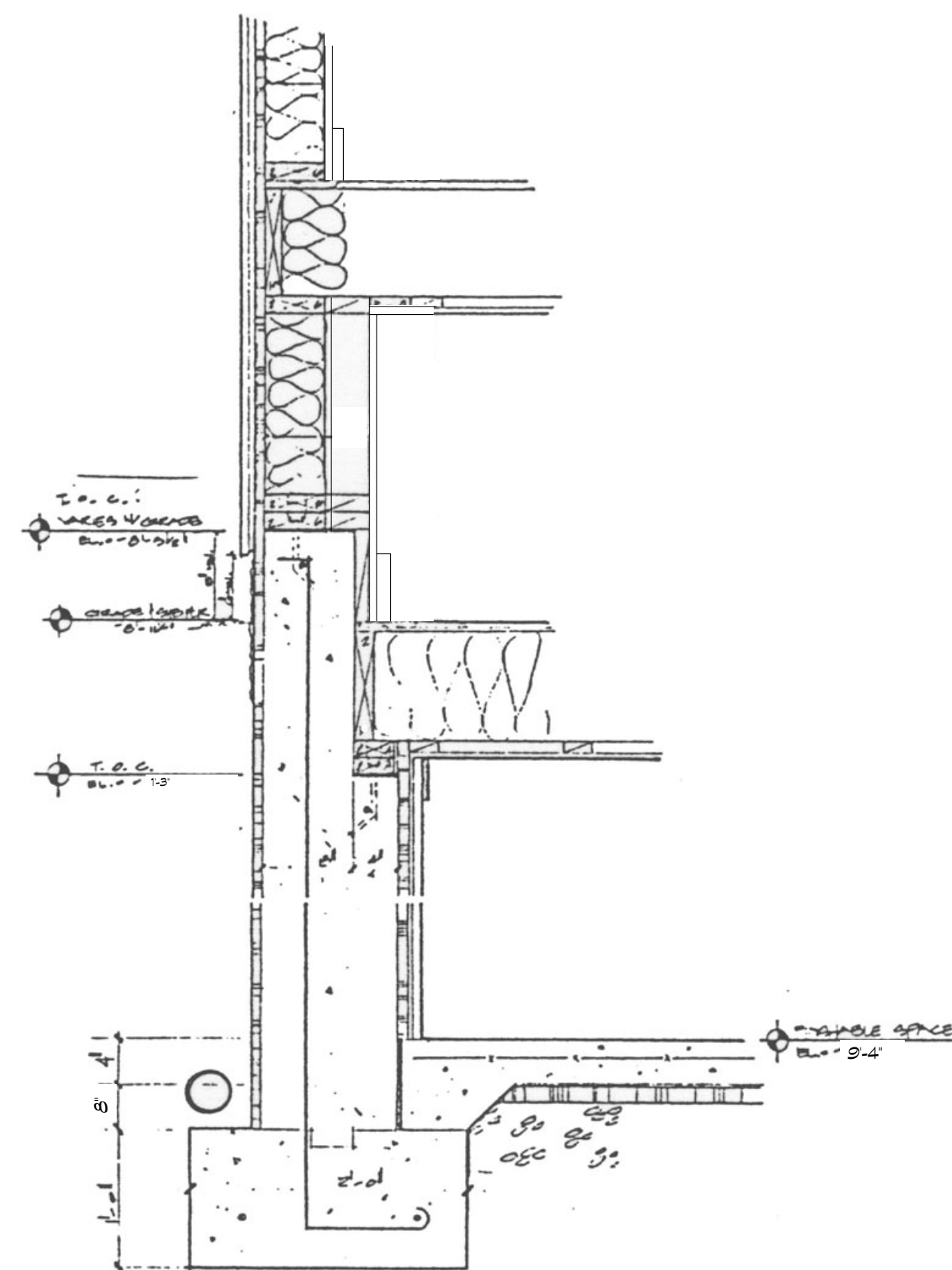
Rear Wall #19 / D11 N.T.S.
